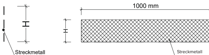
BECOSTRIP ohne Ausschnitte
