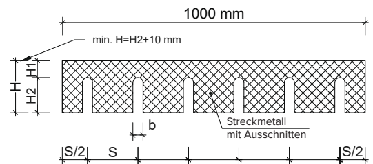
BECOSTRIP mit Ausschnitte
