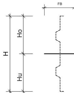
ASF-V Fugenblech H= 150-1200 mm
