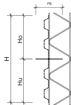
ASF-VG Fugenblech H= 300-2000 mm
