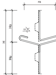
ASF-V Fugenband H= 240-1200 mm
