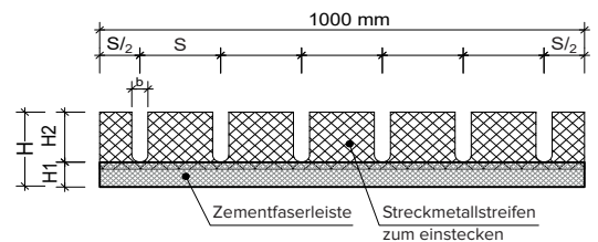
BECOSPACE mit Ausschnitte
