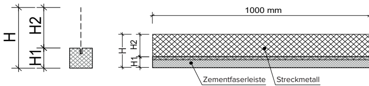
BECOSPACE ohne Ausschnitte
